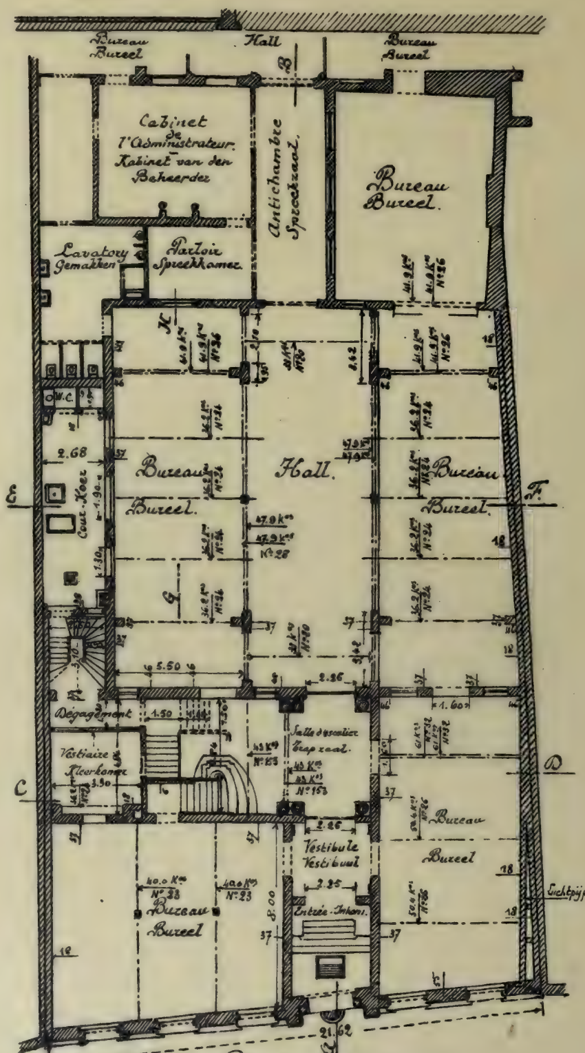
— Plan du rez-de-chaussée — — Plan van gelijkvloers. —
